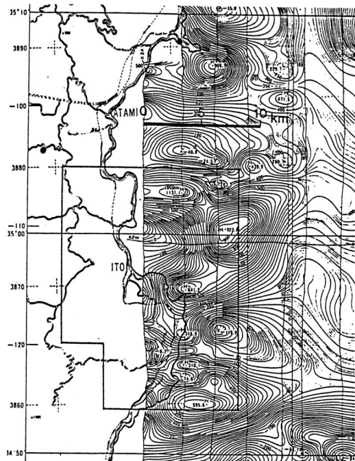
図2. 探査区域と1978年調査の空中磁気図。
