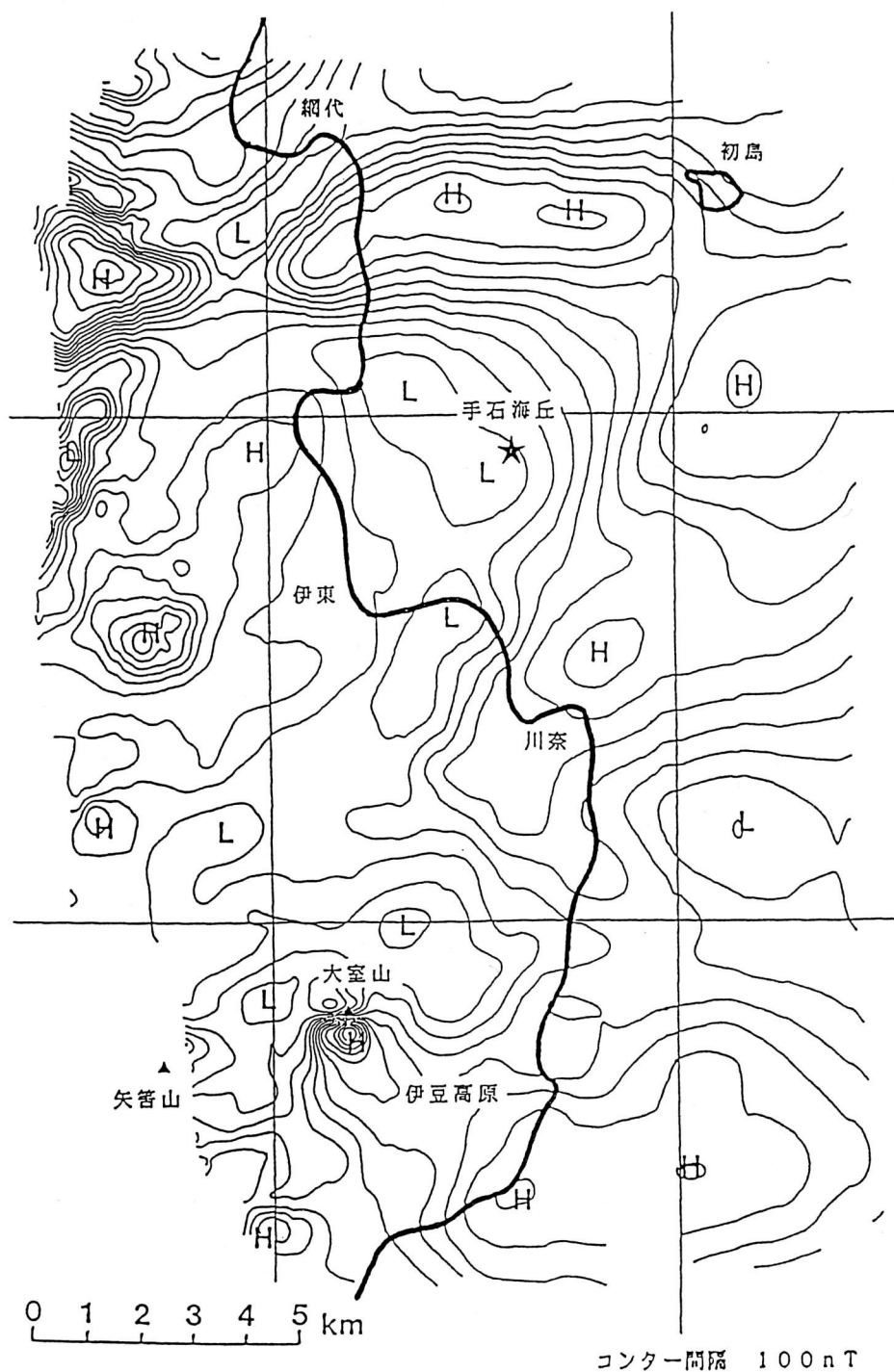
図4. 1989年9月調査による伊豆半島東部地域のIGRF残差空中磁気異常図。 飛行高度は海面上700m (2,300ft) で、南北方向の測線約50本による。
