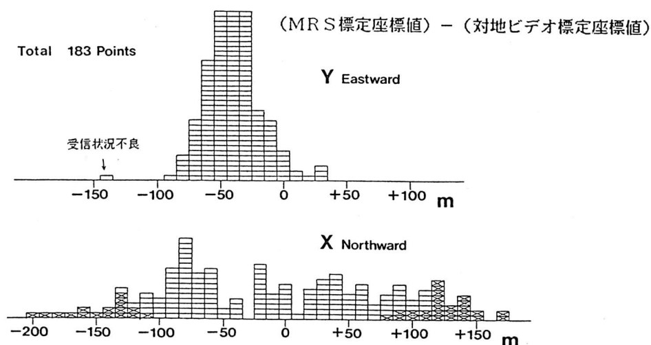
図3. MRS測位と対地ビデオ標定との比較。誤差ベクトルを南北成分と東西成分で表示した。×印は、対地ビデオ装置の時刻ずれが相対的に大きかった特定のフライトに関する比較データ。
